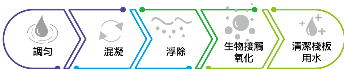
圖、大華金屬廢水處理流程圖
